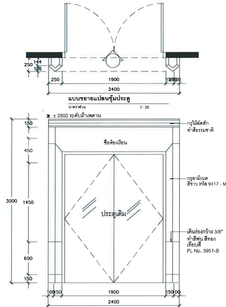
แบบขยายรูปด้าน 35 10-XX
