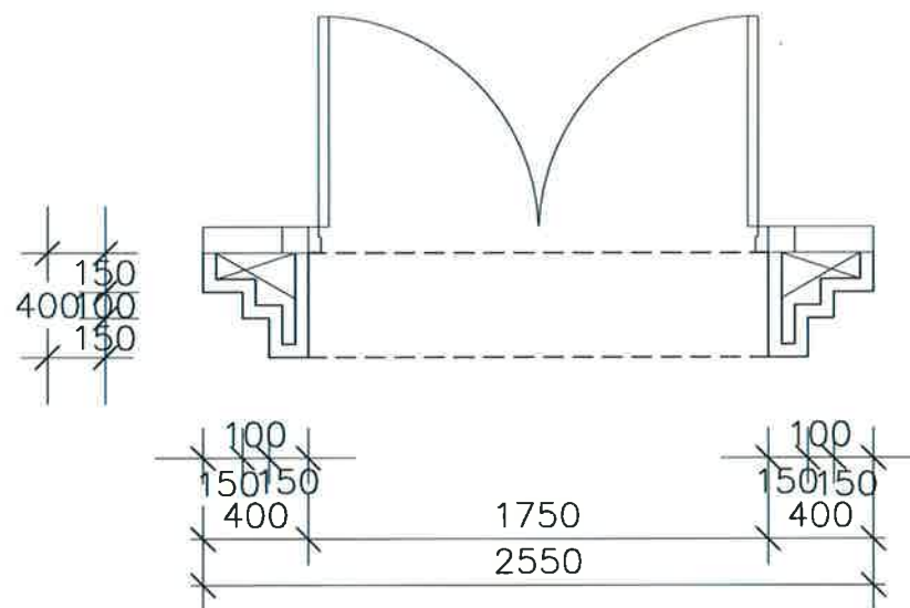
แปลนขยายซุ้มประตูหน้าต่าง
