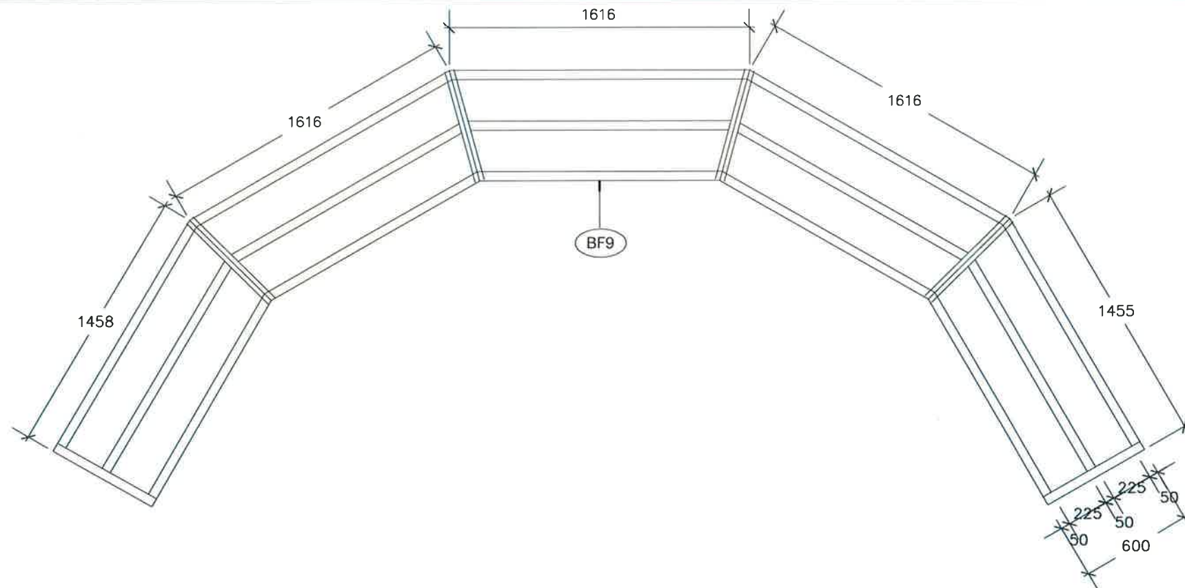
แปลนขยายชุดตู้โสนั่งสือโค้ง 2 ด้าน
